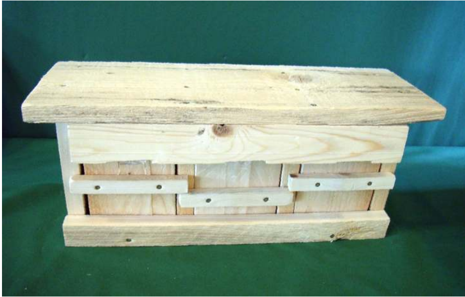
2 Objekte Nistkästen
